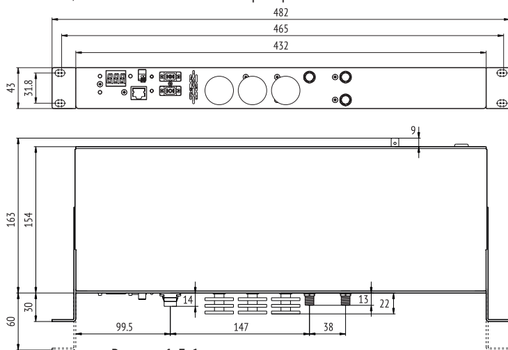
Рисунок 1. Габаритные и установочные размеры
